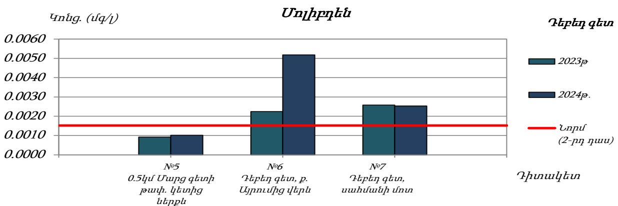
Գծապատկեր 74. Դեբեդ գետի ջրում մոլիբդենի կոնցենտրացիան 2023-2024 թթ.
