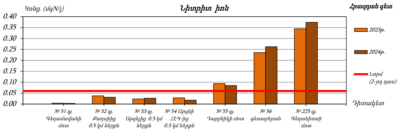
Գծապատկեր 97. Հրազդան գետի ջրում նիտրիտ իոնի կոնցենտրացիան 2023-2024թթ.
