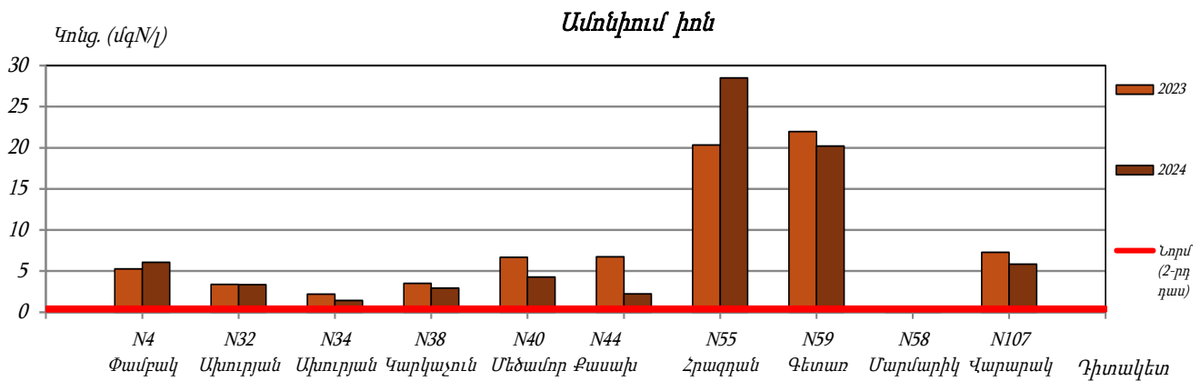
Գծապատկեր 65. Ամոնիում իոնի կոնցենտրացիան կոմունալ-կենցաղային կեղտաջրերով աղտոտված հիմնական գետերում 2023-2024 թթ.
