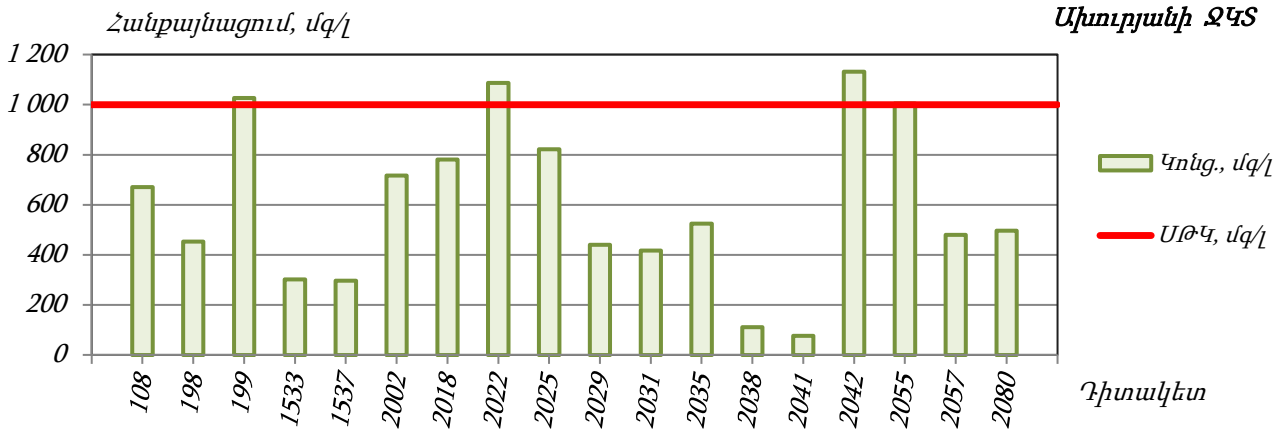
Գծապատկեր 51. Ախուրյանի ՋԿՏ-ի ստորերկրյա ջրերի դիտակետերի հանքայնացումը
