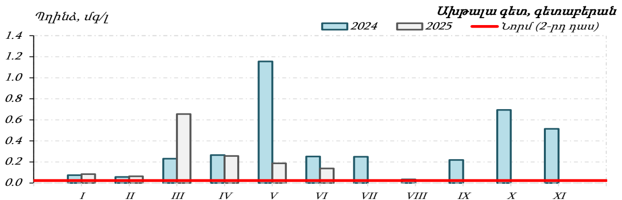
Գծապատկեր 42. Ախթալա գետում պղնձի կոնցենտրացիաները
