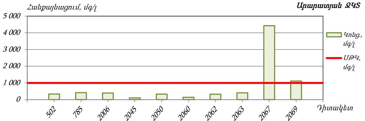
Գծապատկեր 62. Արարատյան ՋԿՏ-ի ստորերկրյա ջրերի դիտակետերի հանքայնացումը
