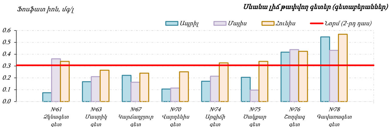
Գծապատկեր 62. Սևանա լիճ թափվող գետերի գետաբերաններում ֆոսֆատ իոնի կոնցենտրացիաների փոփոխությունները
