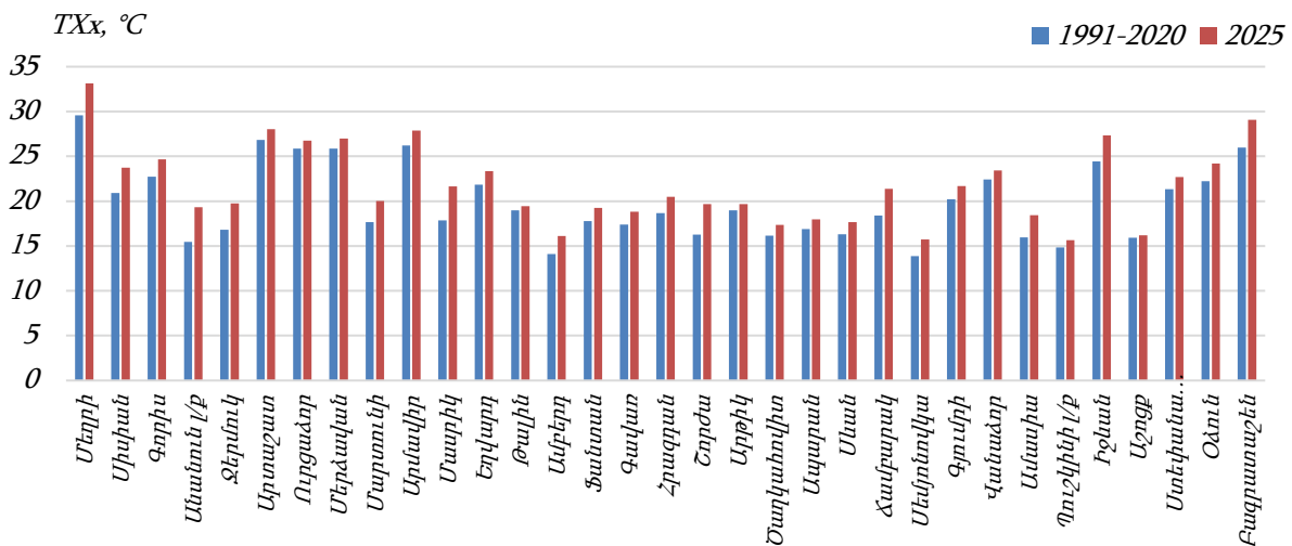
Գծապատկեր 3. Օրական առավելագույն ջերմաստիճանների արժեքները 2025թ. զարնանը
