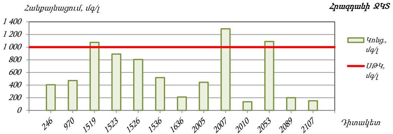
Գծապատկեր 62. Հրազդանի ՋԿՏ-ի ստորերկրյա ջրերի դիտակետերի հանքայնացումը
