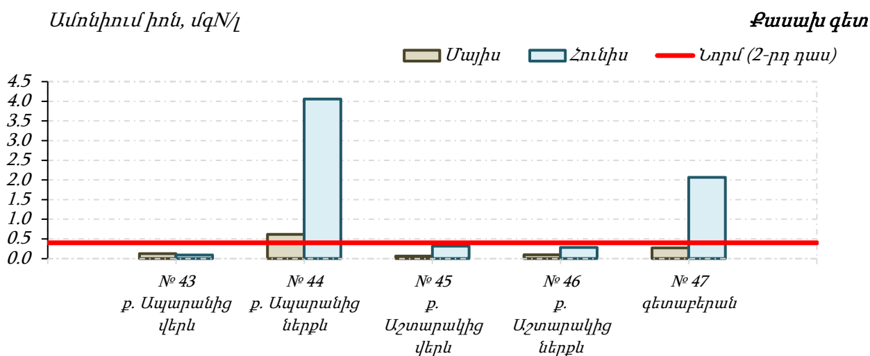
Գծապատկեր 52. Քասախ գետում ամոնիում իոնի կոնցենտրացիաների փոփոխությունները Ամոնիում իոն, մգN/լ
